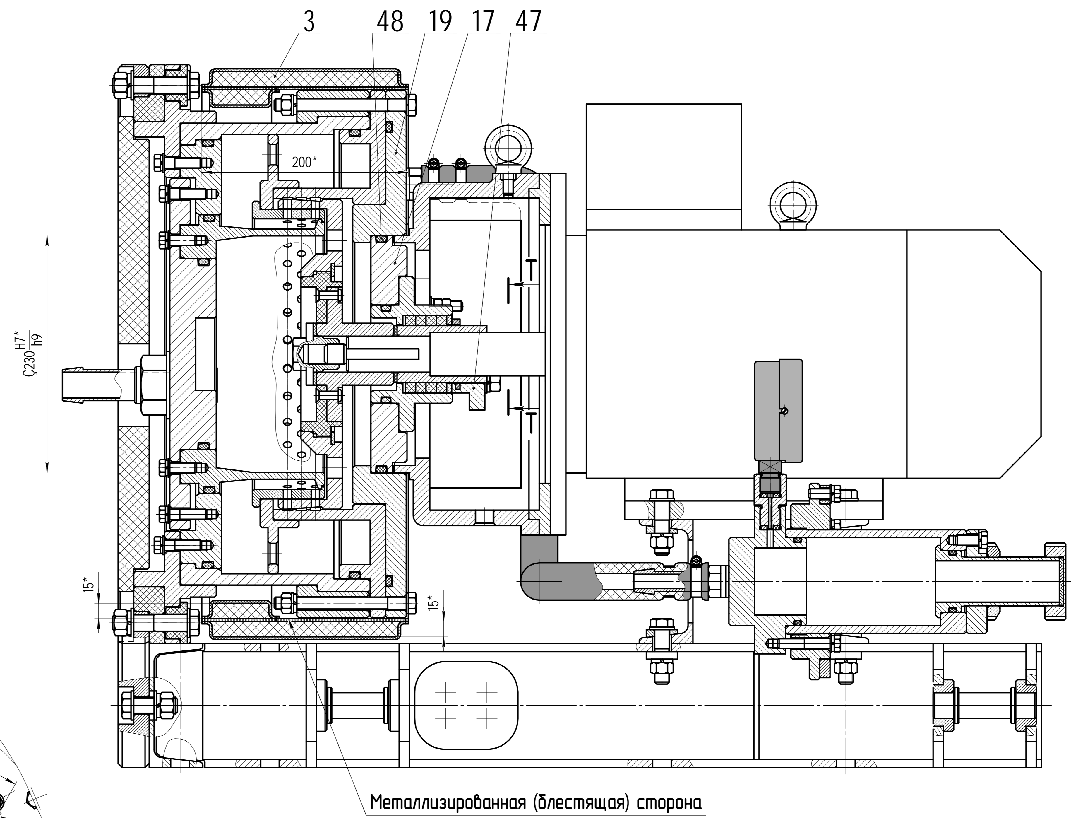
Рис. 2. (ТРКГ.00.000-01), остальное смотри Рис. 1 (листы 1, 2)
